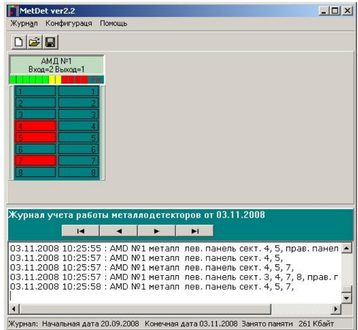
Рис. 6 – Основное окно программы «Met Det Control ver.2.2»
